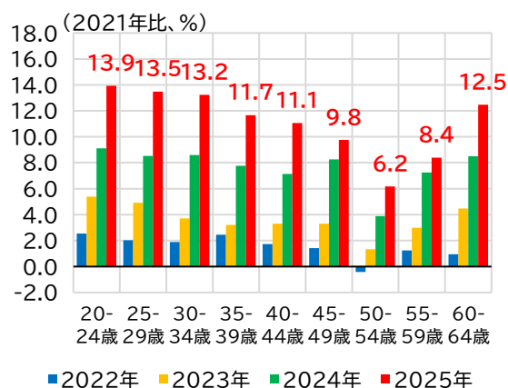
図2 年齢階級別の所定内給与：累積
